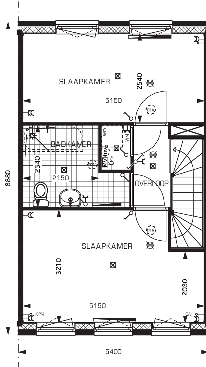
2 E VERDIEPING TYPE P Bouwnummer P: 25
