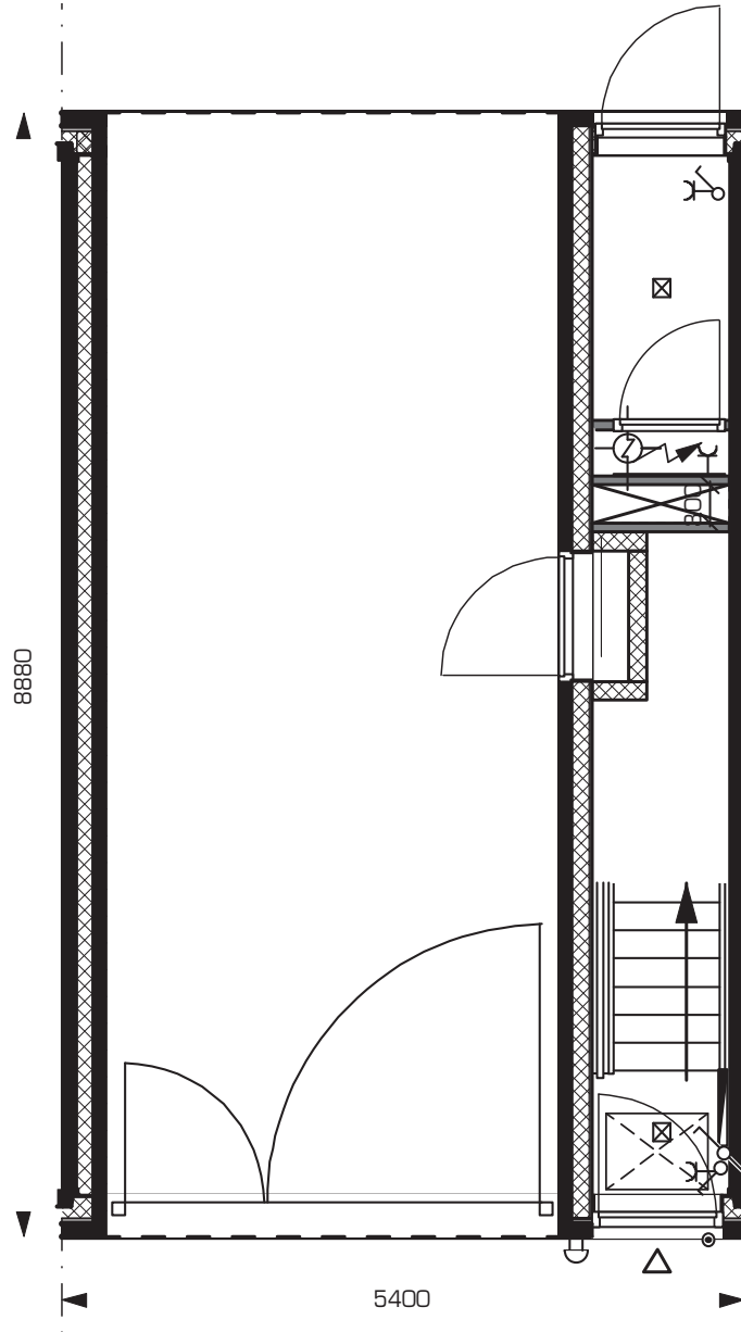
BEGANE GROND TYPE P
