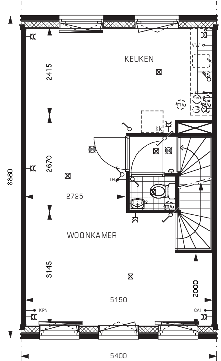
1 E VERDIEPING TYPE P
